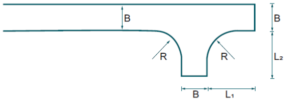
■ Figur 4.29 Vendeplads udformet som asymmetrisk hammerhoved, principskitse.
