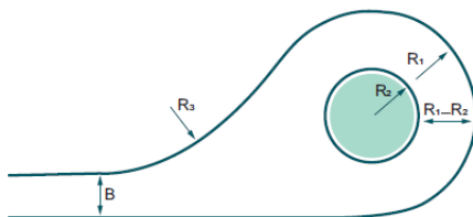
■ Figur 4.25 Cirkelformet vendeplads, principskitse.
