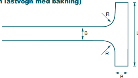
■ Figur 4.27 Vendeplads udformet som symmetrisk hammerhoved, principskitse.
