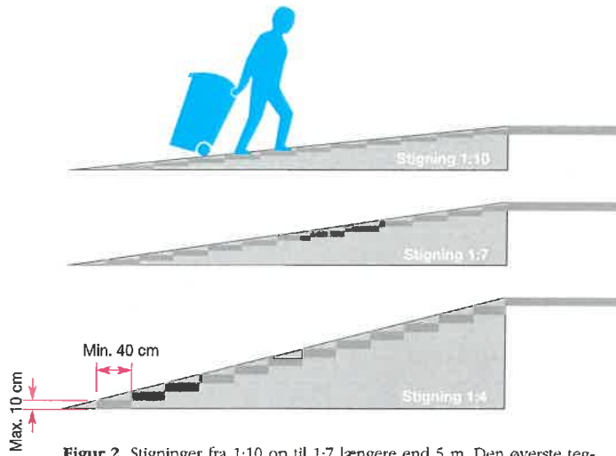
Figur 2. Stigninger fra 1:10 op til 1:7 længere end 5 m. Den øverste tegning illustrerer fx en hædning på 1 m over 10 m. Den nederste tegning illustrerer fx en hædning på 2 m over 8 m.
