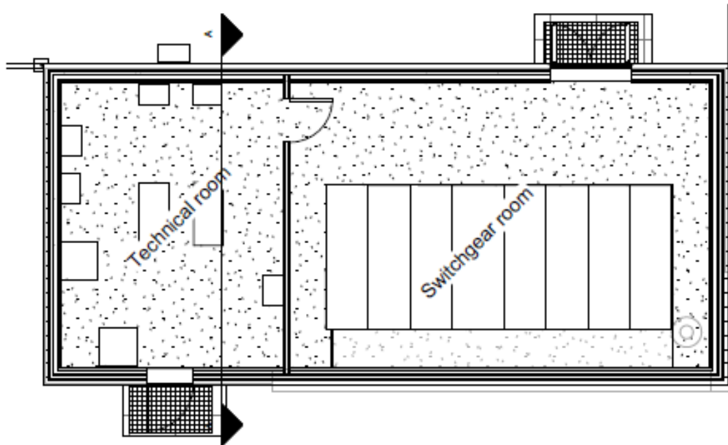
Plantegning
