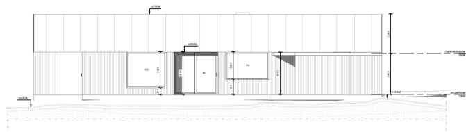
FACADE MOD SYD 1 : 50
