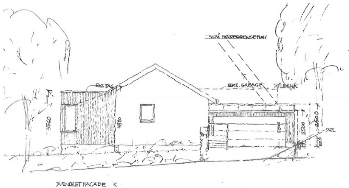
FACADE MOD SYDVEST 1:100
