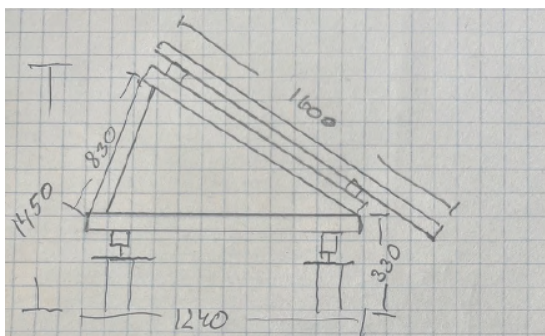
Figur 2: Skitse af solcelleanlægget
