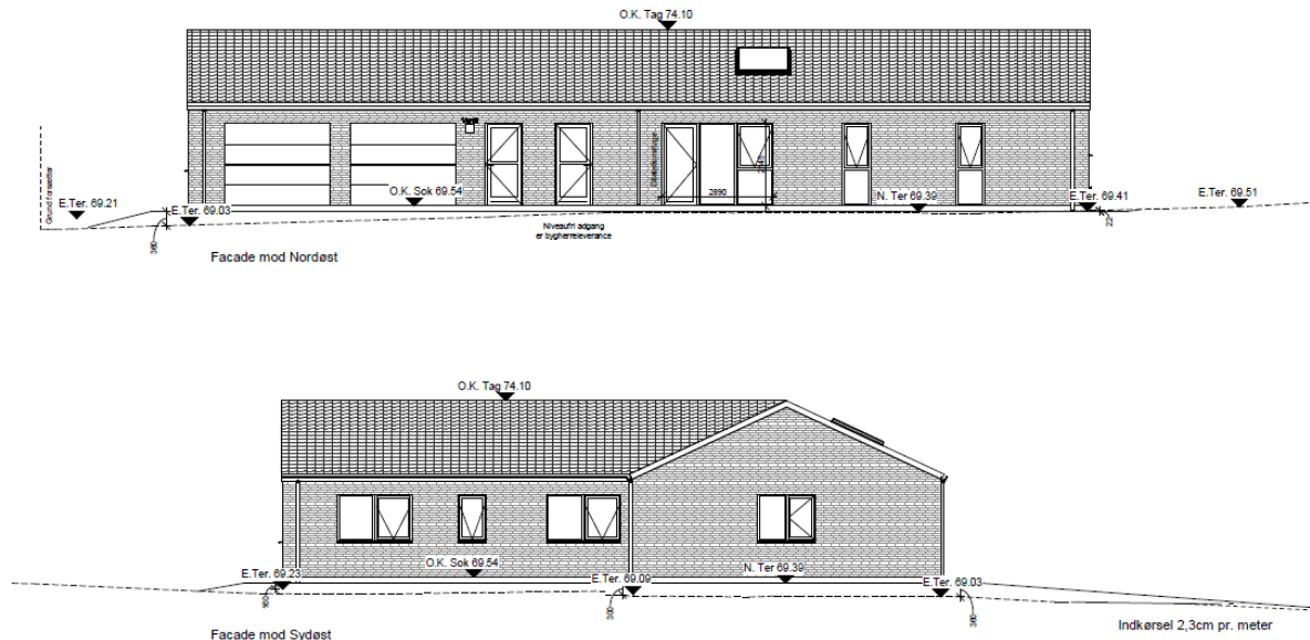
Facadetegninger
