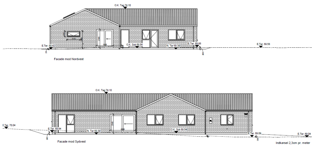
Facadetegninger
