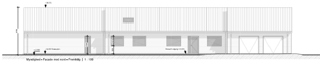
Myndighed - Facade mod nord - Fremtidig | 1 : 100
