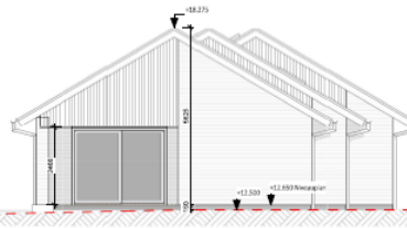
Myndighed - Facade mod øst - Fremtidig | 1 : 100
