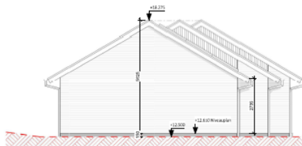
Myndighed - Facade mod vest - Fremtidig | 1 : 100
