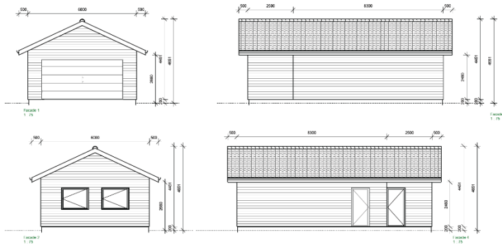
Facader af byggeriet på Marienborgvej 2, 9510 Arden
