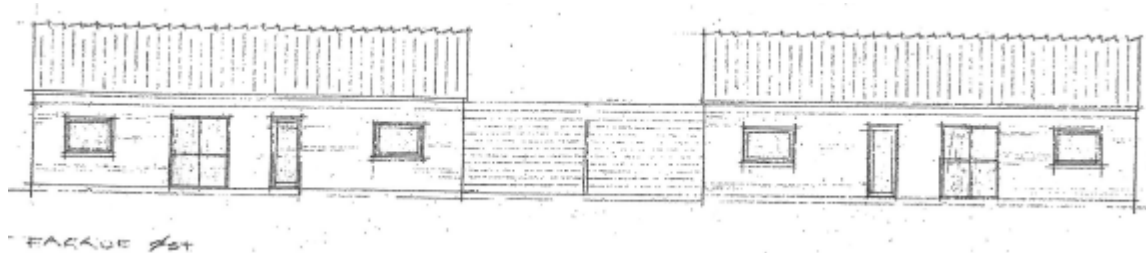
Fig. 3 Facadetegning af dobbelthuset mod øst
