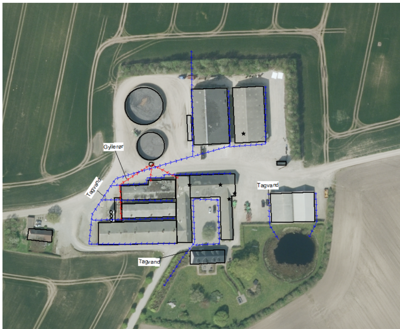
Afløbsplan
