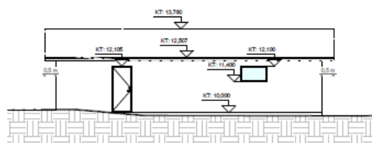
Øst - Fremtidig. 1 : 100
