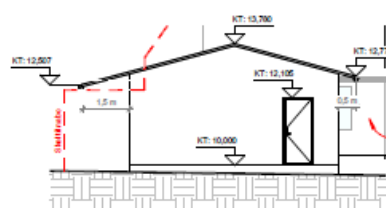
Nord - Fremtidig. 1 : 100
