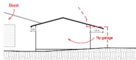
Syd - Fremtidig. 1 : 100
