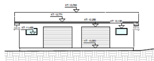
Vest - Fremtidig. 1 : 100
