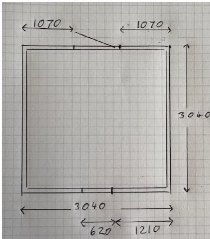
Figur 5: Plantegning for legehus
