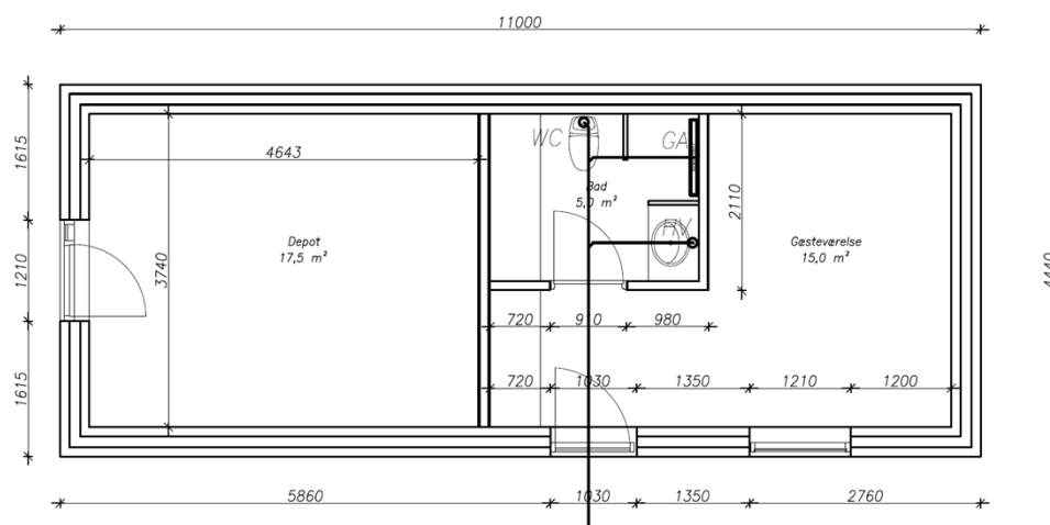
Figur 1: Plantegning
