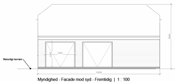
Facadetegninger
