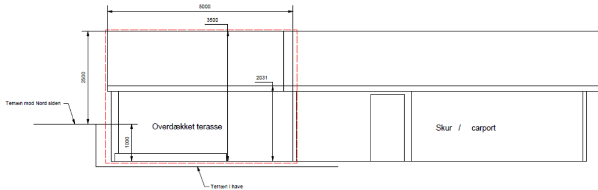
Facade syd
