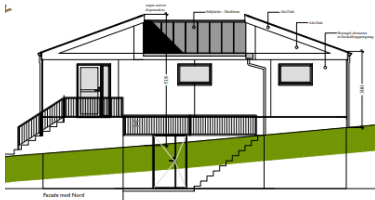
Facade nord
