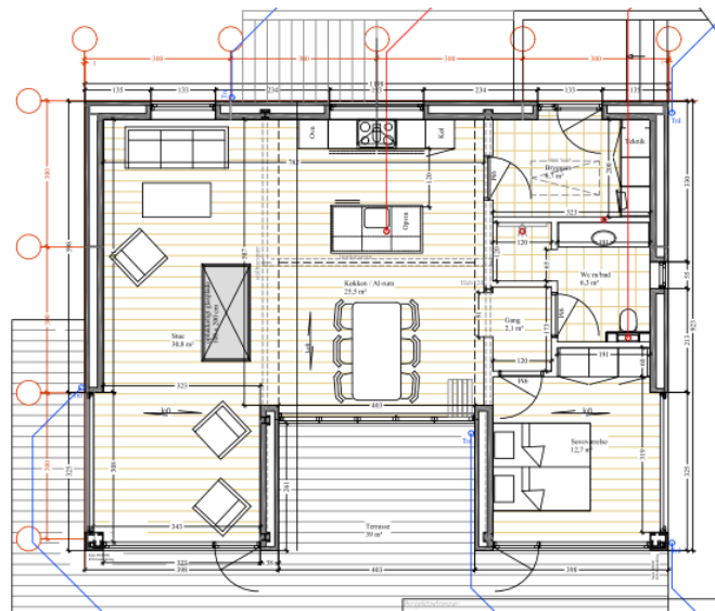
Stueplan
