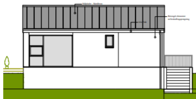
Facade øst
