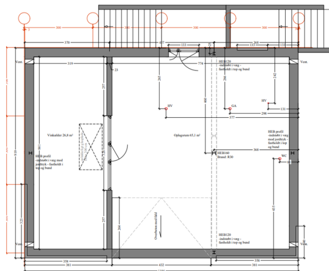
Kælderplan
