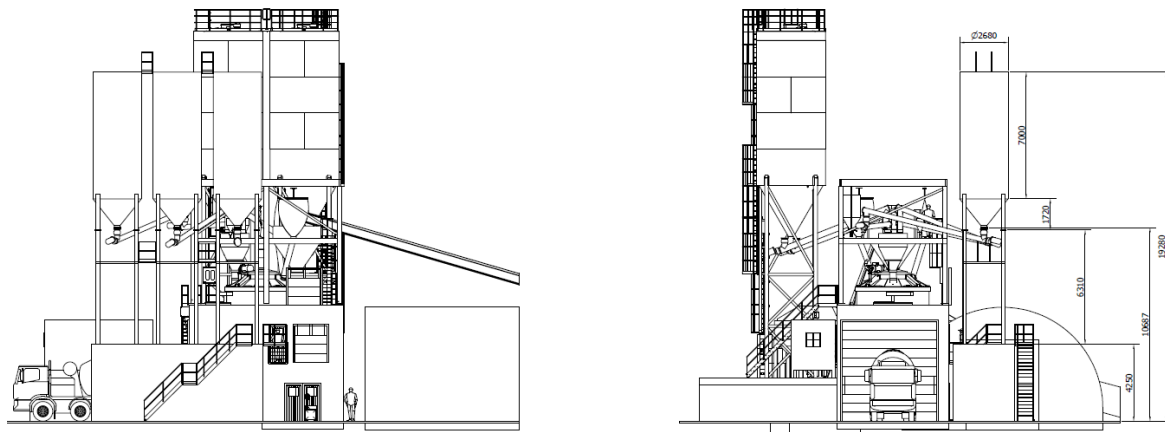
Opstalter af siloerne set fra vest (til venstre) og fra nord (til højre)
