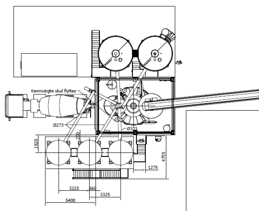
Situationsplan med siloernes placering ved eksisterende byggeri
