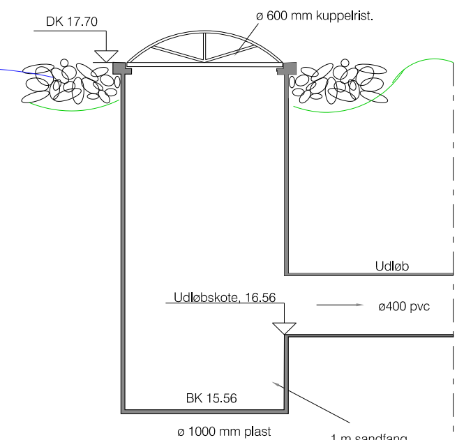
SNIT A-A AF NØDOVERLØB 04GR034
