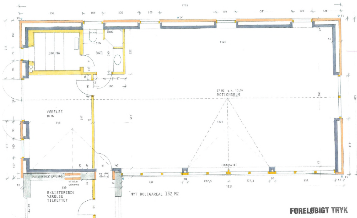
Figur 4: Stueplan
