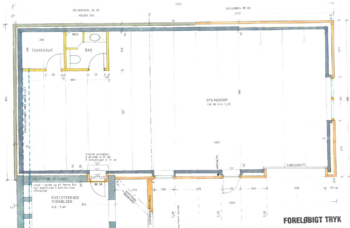
Figur 3: Kælderplan
