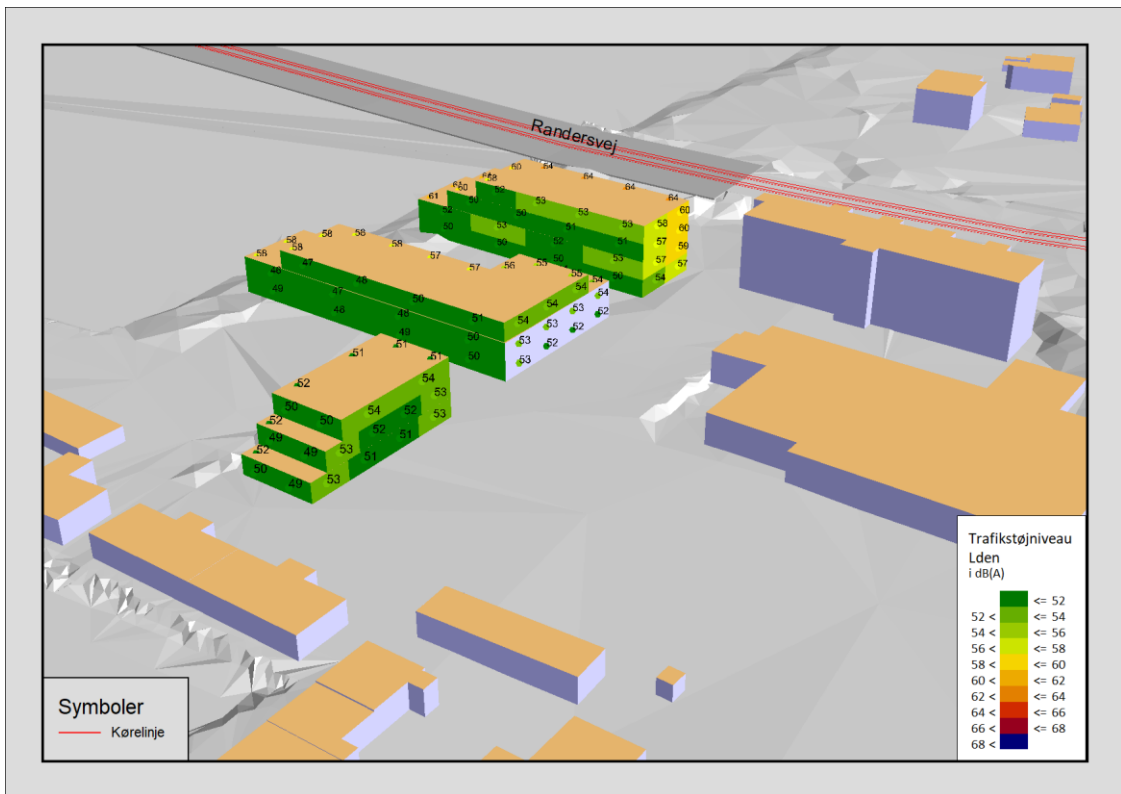
Figur 3b. Facadeniveauer set fra nord.
