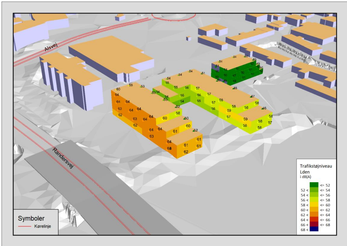
Figur 3a. Facadeniveauer set fra syd.
