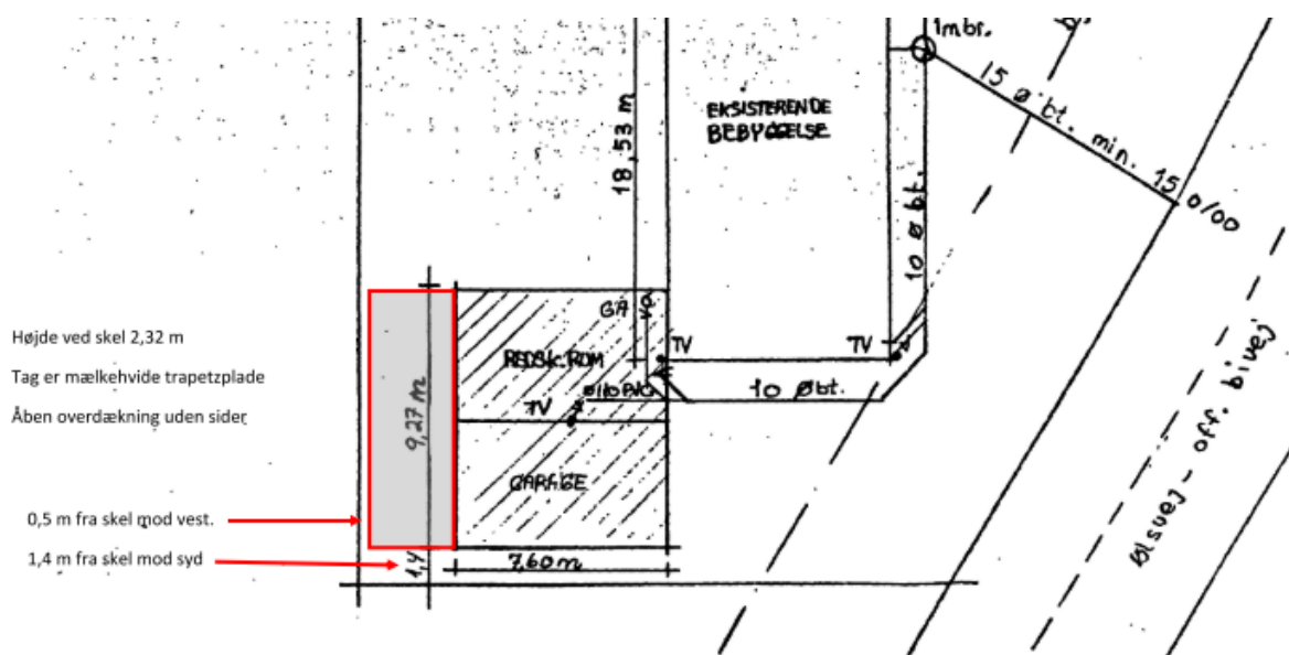
Figur 1: Situationstegning over Ølsvej 30, 9500 Hobro, som viser bygningernes placering på grunden.
