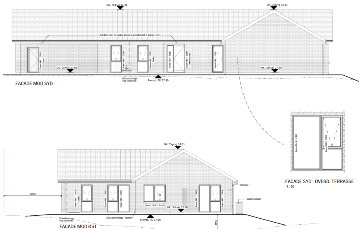
Figur 3: Facadetegninger, syd og øst
