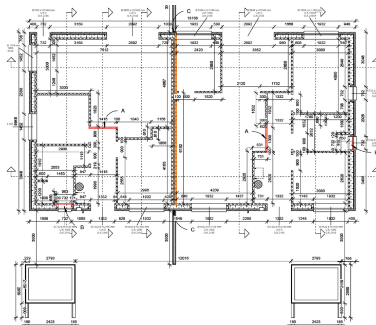
Plantegning af byggeriet
