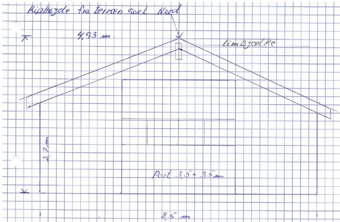
Figur 4: Nordfacade med port
