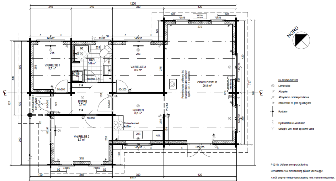
Plantegning
