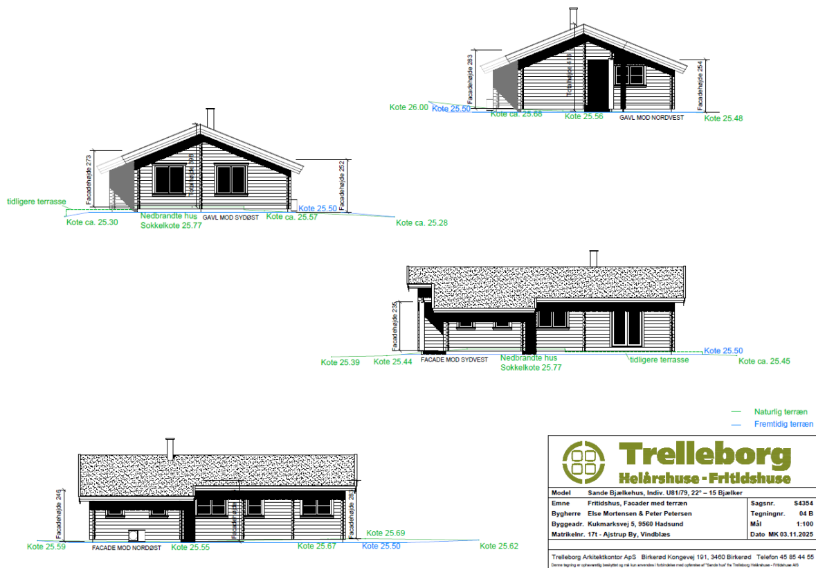
Facadetegninger
