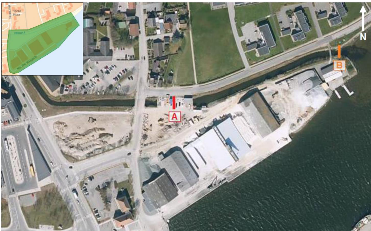
Figur 4.1 Placering af sluseløsninger. Løsning A (rød). Løsning B (orange). Sikringsområdet (grøn).
